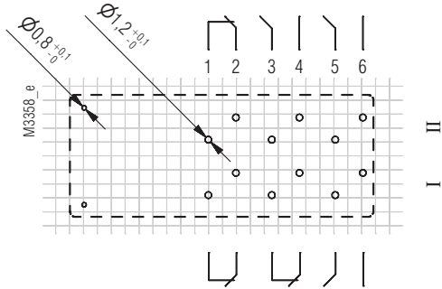
OA 5622.18/___W7 3NO / 3NC
