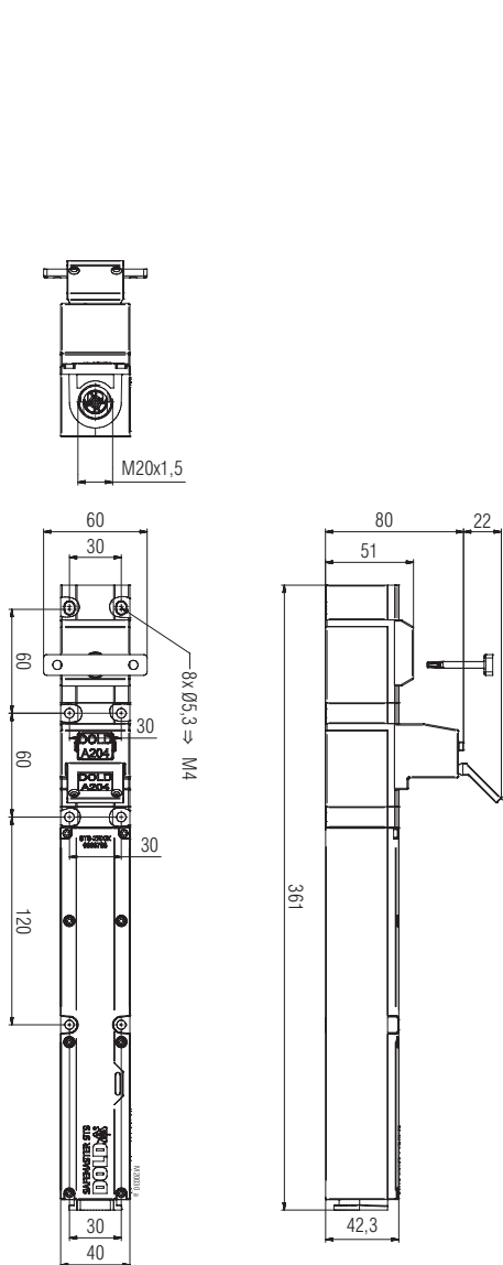
YRX10BM/K Freimaßtoleranzen ± 2%
