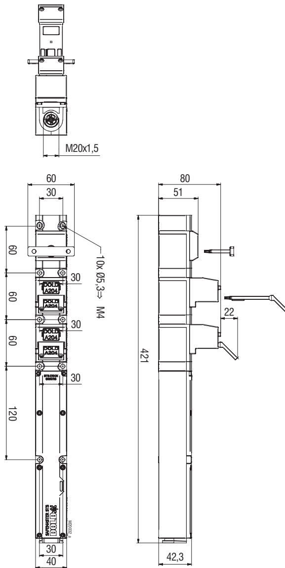
YRX11BM/K Freimaßtoleranzen ± 2%
