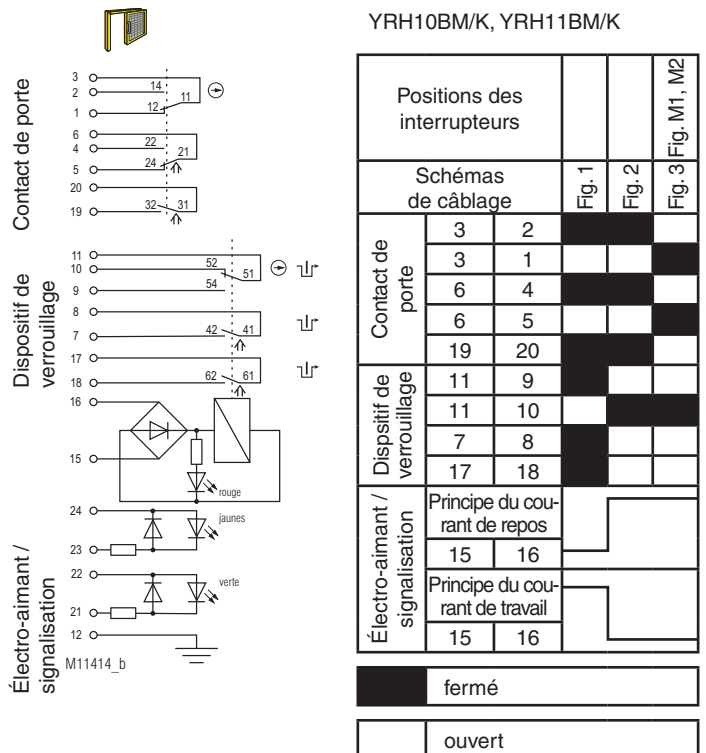
Fig. 3 : Gâche à l'état désactivé: Électro-aimant déverrouillé, clé insérée
